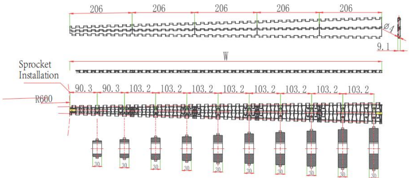
sprocket P213
